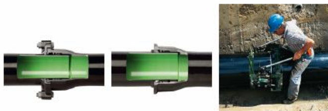
Buitenliggende trekvast koppeling Binnenliggende trekvast koppeling
